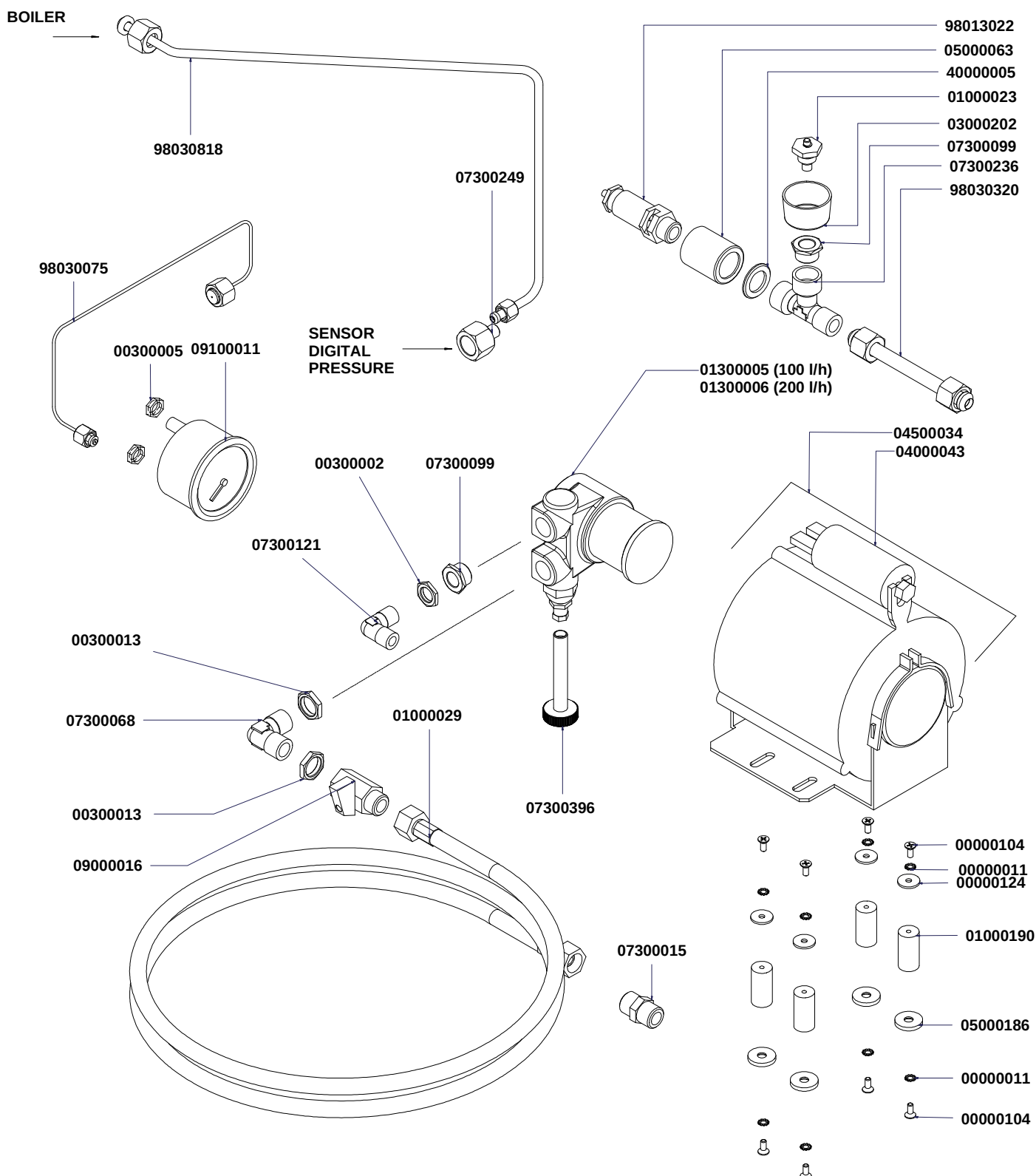
Componenti idraulici carico Hydraulic Components load
